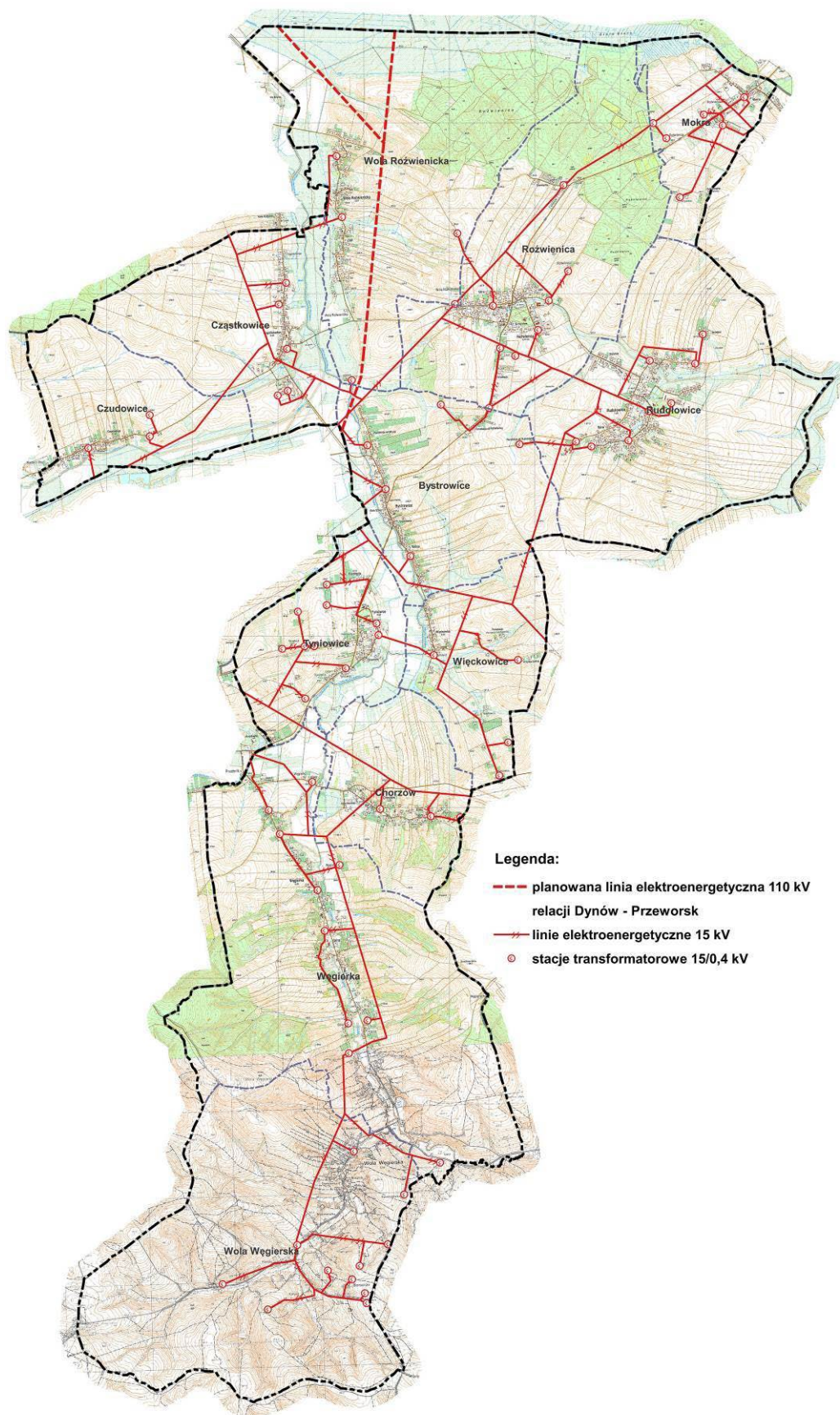
schemat 7- Lokalizacja infrastruktury elektroenergetycznej na terenie gminy Rożwnica
